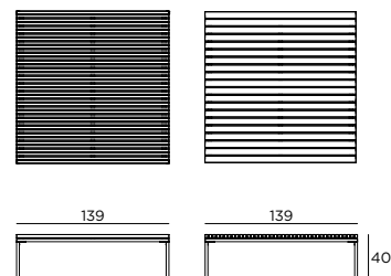
LOUNGETISCH 140/140 LOUNGE TABLE 140/140
