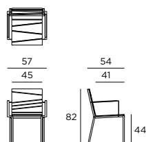
STUHL MIT ARMLEHNE CHAIR WITH ARMREST
