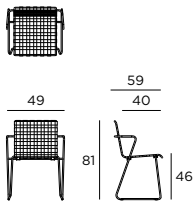
STUHL BELT MIT ARMLEHNE CHAIR BELT WITH ARMREST
