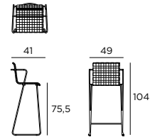
BARSTUHL BELT MIT ARMLEHNE BARSTOOL BELT WITH ARMREST
