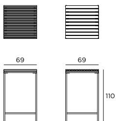
STEHTISCH HIGH TABLE
