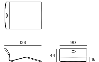
LOUNGER ZWEISITZER DOUBLE LOUNGER
