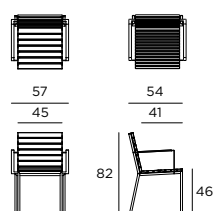
STUHL MIT ARMLEHNE CHAIR WITH ARMREST
