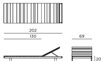
HOLZ SONNENLIEGE WOODEN SUNLOUNGER
