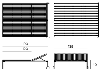
DOPPELLIEGE DOUBLE SUNLOUNGER
